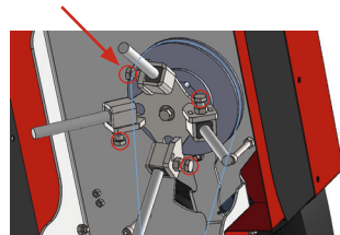
(Abb. 5 - Drahtzöpfe wechseln)
